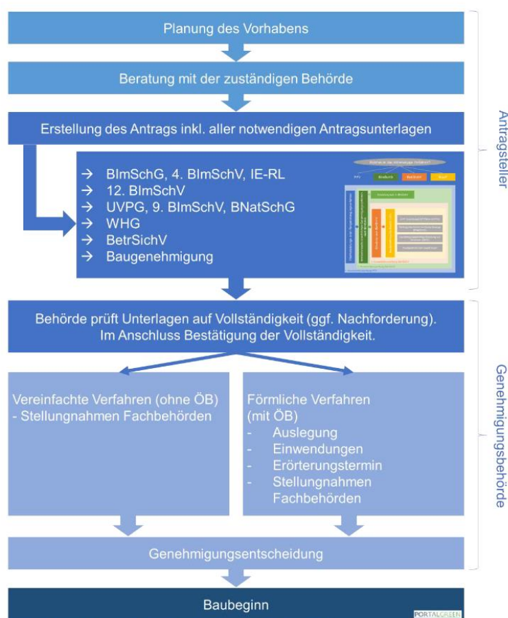
Abb. 2.3: Ablauf BImSchG-Verfahren - Urheber: DBI
